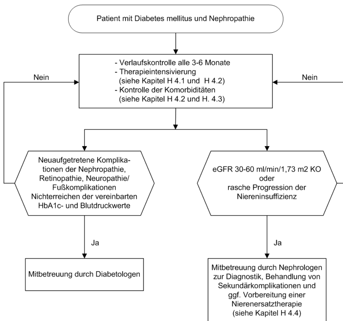
Algorithmus 3: Schnittstellendefinition
